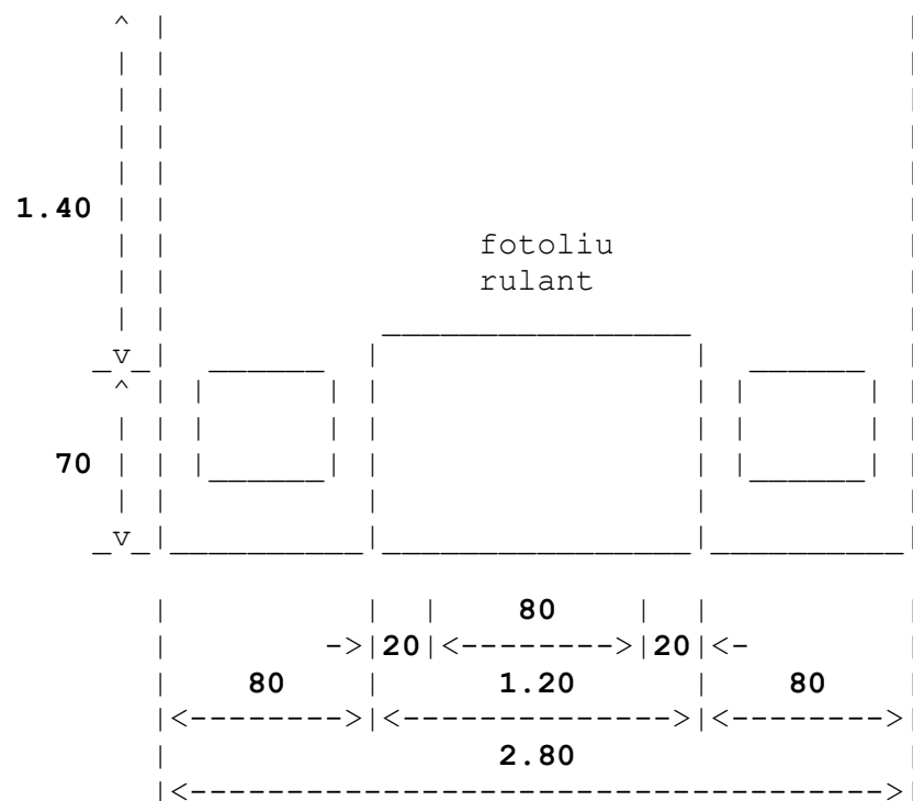
Fig. VII.4.b. - Spații necesare la masă și pentru circulația utilizatorilor de fotoliu rulant
