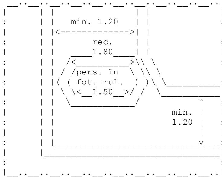
Fig. V.3. - Intersecție de coridoare
