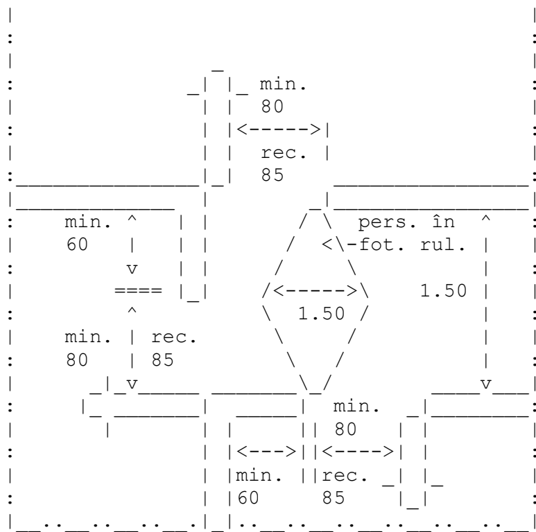
Fig. V.6. - Amplasarea ușilor la un coridor înfundat
