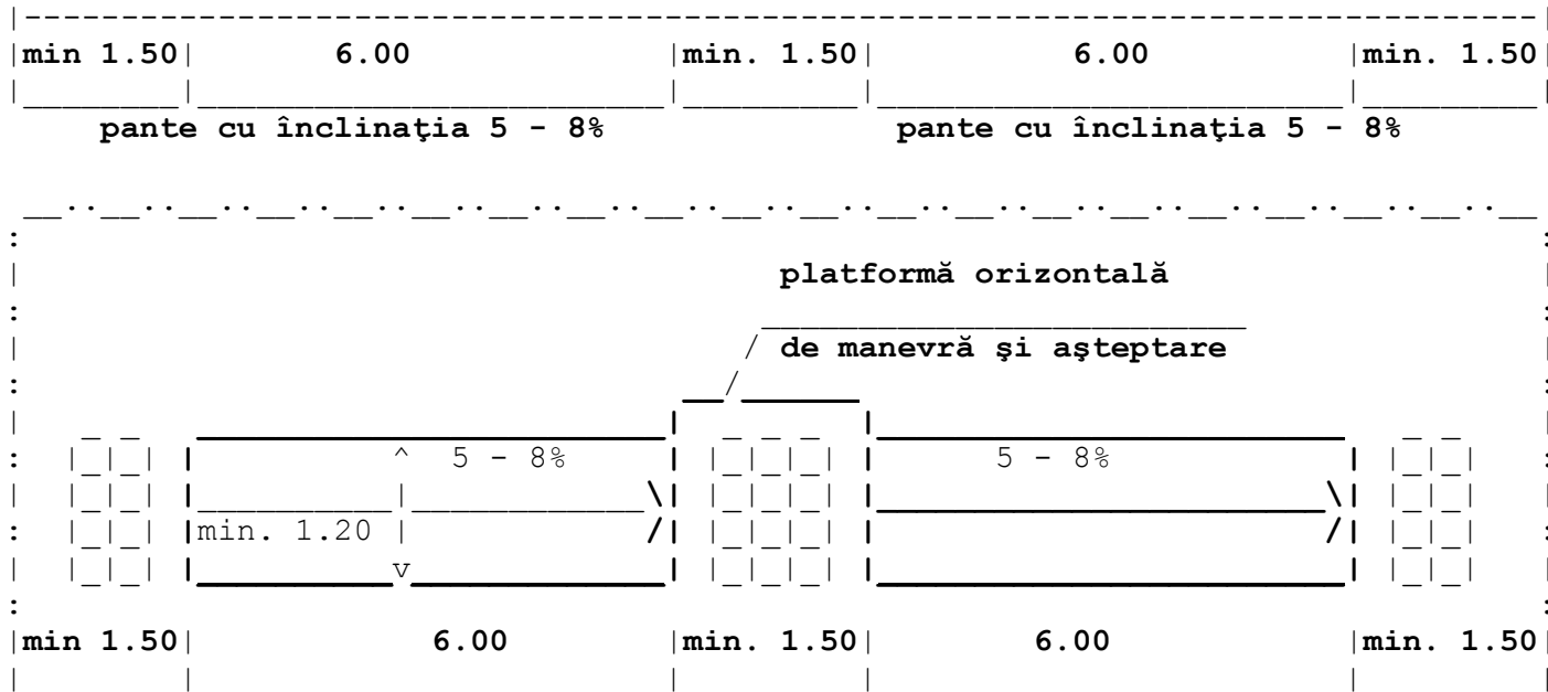
Fig. V.30. - Conformarea rampelor (idem Fig. IV.3.)
