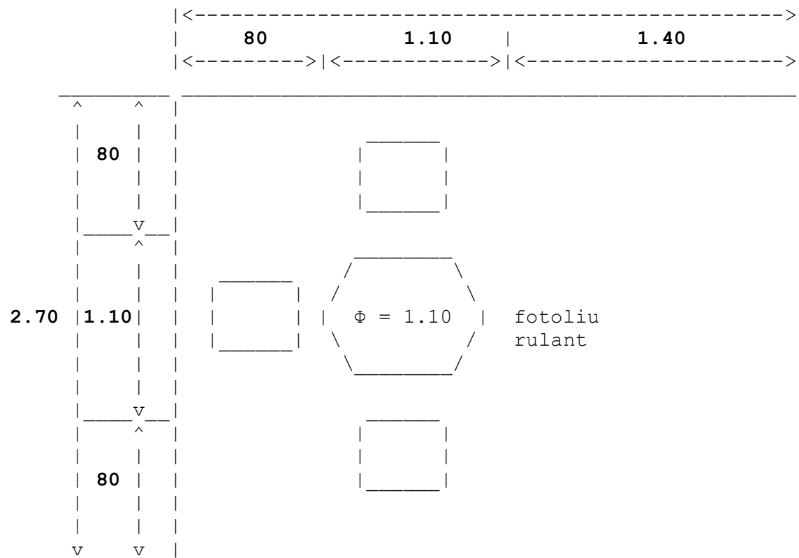
Fig. VII.4.a. - Spații necesare la masă și pentru circulația utilizatorilor de scaun rulant
