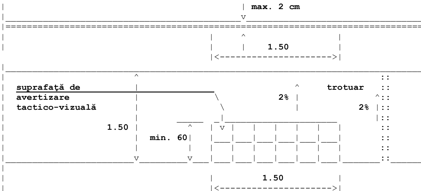
Fig. IV.9. - Rampă de acces între trotuar înclinat și carosabil
