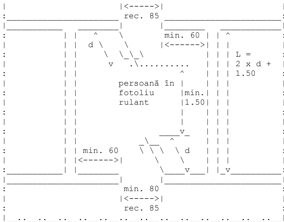
Fig. V.22. - Dimensionarea spațiului pentru deschiderea ușilor către interior
