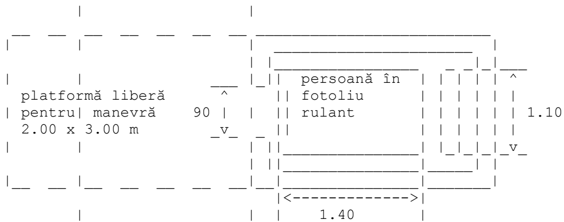
Fig. V.14. - Ascensor pentru o persoană utilizatoare de fotoliu rulant, cu însoțitor (dimensiuni minime ale cabinei)
