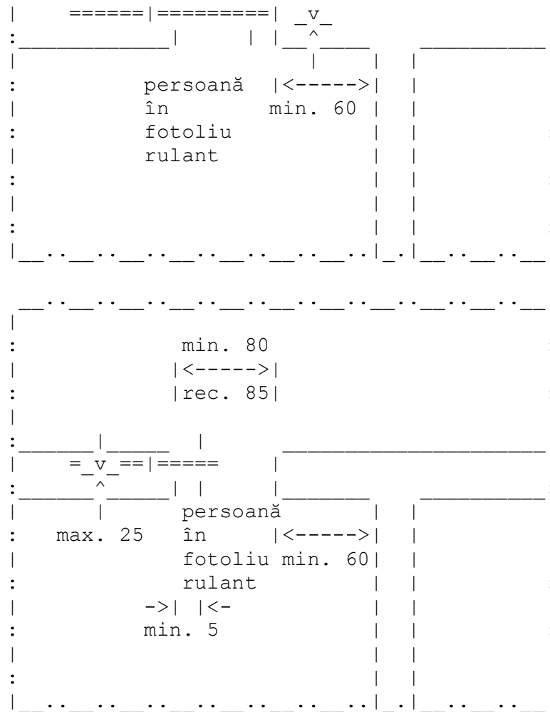
Fig. V.20. - Uși interioare culisante
