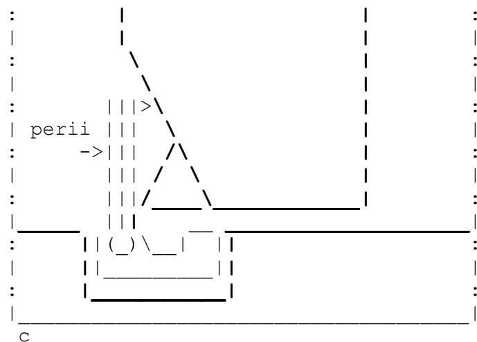
Fig. V.26. - Conformarea pragurilor la ușile interioare a. soluție cu ghidaj îngropat pentru uși culisante b. soluție cu lamelă ridicătoare prin apăsarea clanței c. soluție cu clapetă ridicătoare prin închiderea ușii
