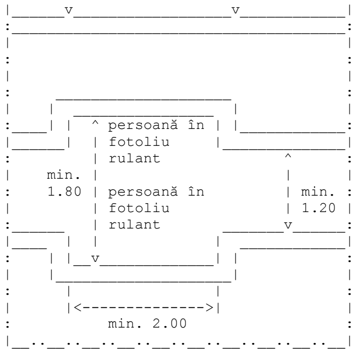
Fig. V.1. - Buzunare la coridoare
