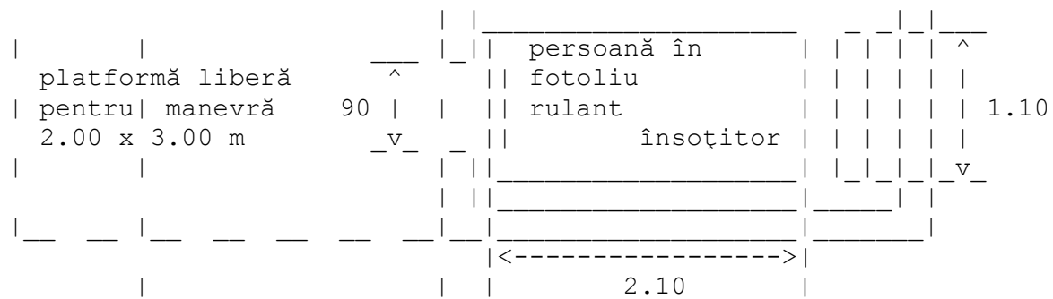
Fig. V.17. - Ascensor pentru o persoană utilizatoare de fotoliu rulant și însoțitorul său
