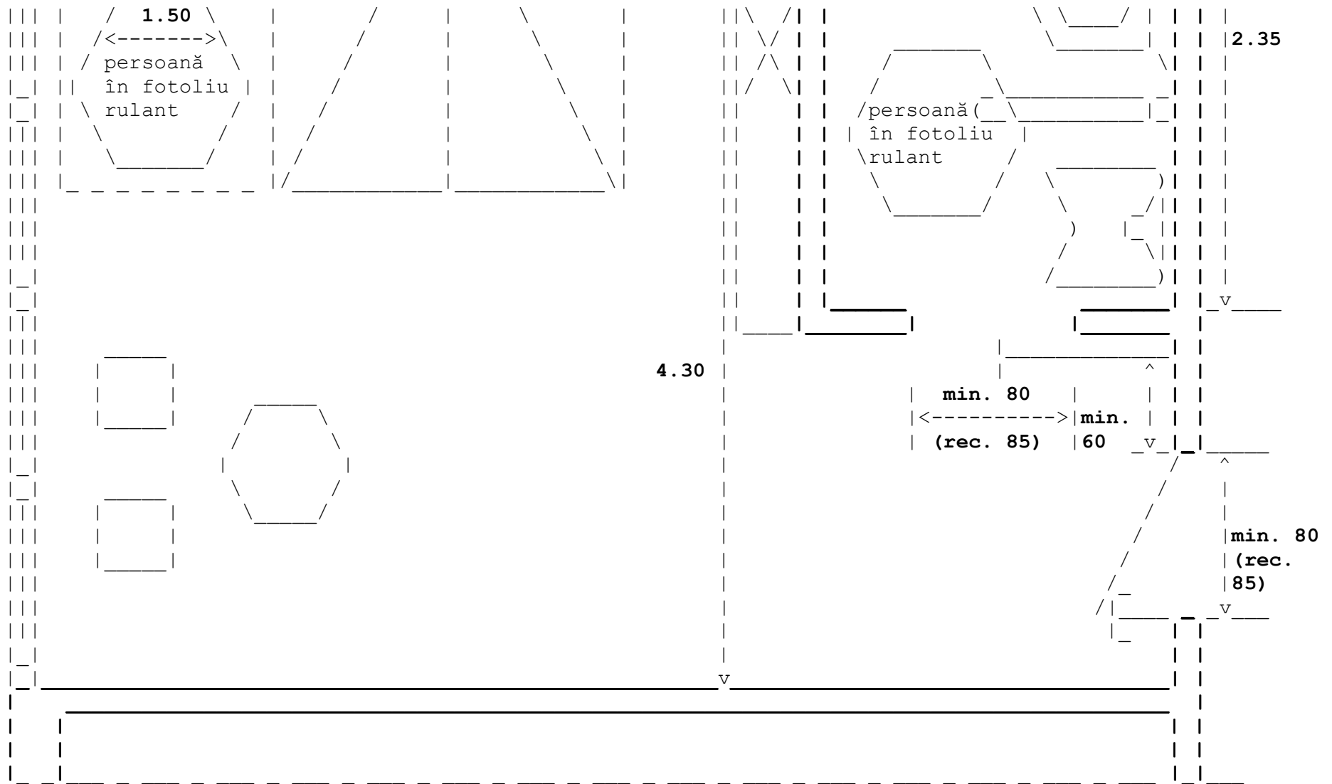
Fig. VII.6. - Schemă de amenajare a unei camere de hotel cu pat dublu
