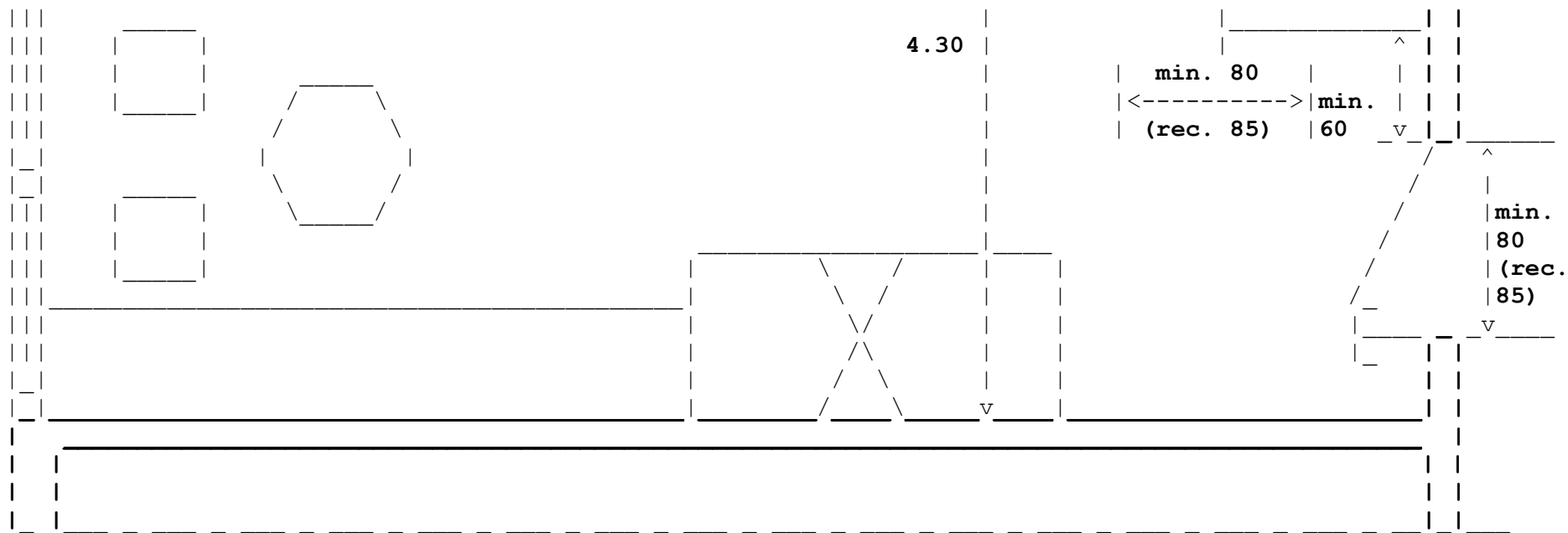
Fig. VII.5. - Schemă de amenajare a unei camere de hotel cu două paturi
