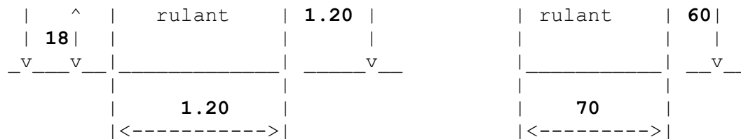
Fig. III.3. - Dimensiuni ale fotoliului rulant - persoane adulte (a se vedea SR EN 12183, SR EN 12184)
