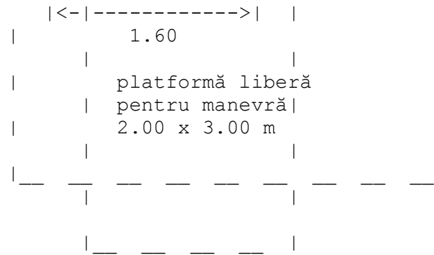
Fig. V.18. - Ascensor cu acces pe două laturi adiacente
