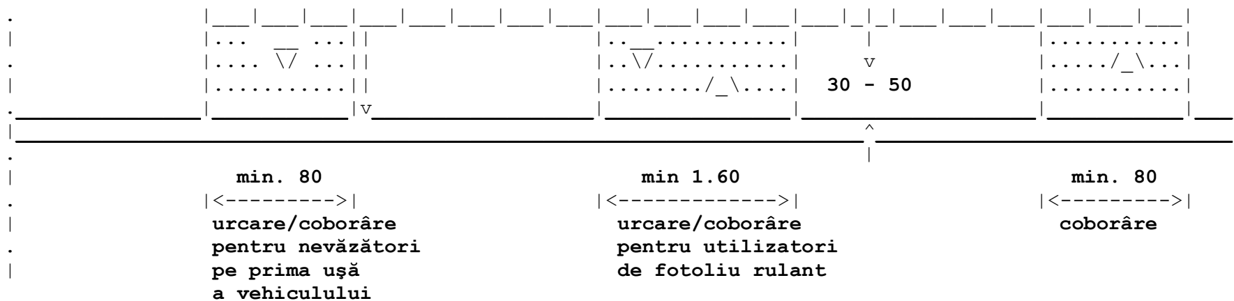
Fig. IV.16. - Stație pentru transport în comun urban
