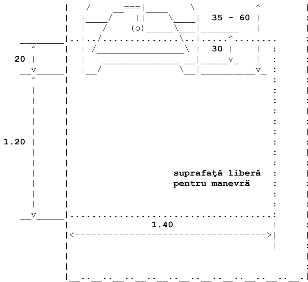
Fig. V.36. - Lavoar conformat și echipat pentru persoane cu handicap
