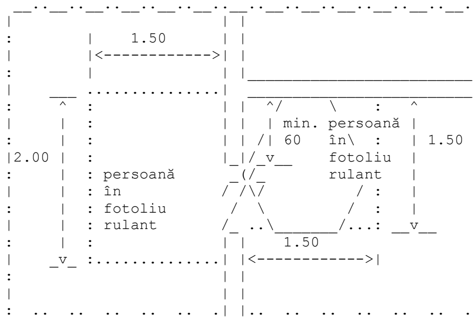
Fig. V.21. - Spațiu de manevră lângă ușă
