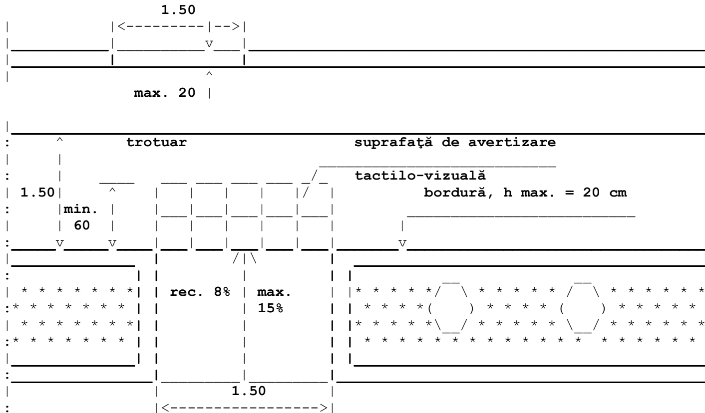
Fig. IV.10. - Rampă de acces între trotuar și carosabil cu bandă de spațiu verde
