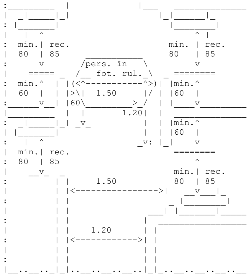
Fig. V.5. - Amplasarea ușilor pe parcursul unui coridor
