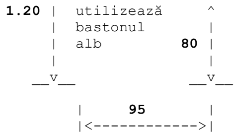
Fig. III.9. - Dimensiuni antropometrice pentru persoane adulte care utilizează bastonul alb
