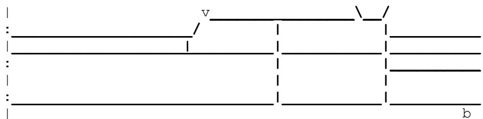
Fig. V.25. - Conformarea pragurilor la uşile către exterior a. soluţie cu rigolă având grătar cu ochiuri < 1,5 cm b. soluţie cu prag cu înălţare
