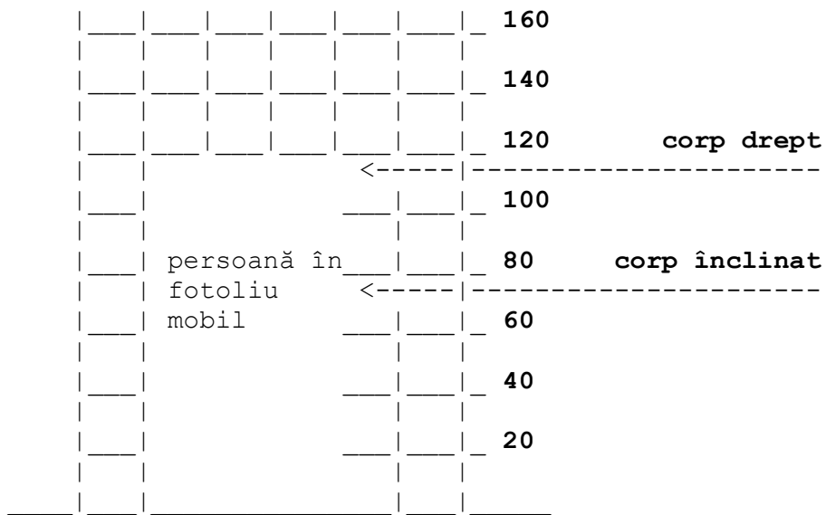
Fig. III.6. - Dimensiuni antropodinamice (în cm) pentru utilizatori ai fotoliului rulant - persoane adulte. Vedere laterală
