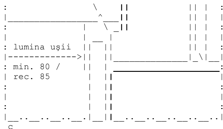
Fig. V.27. - Conformarea balamalelor pentru adaptarea unor goluri de uşi existente
