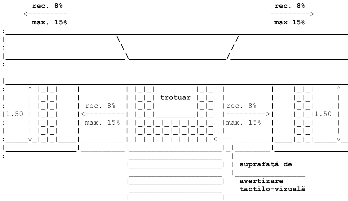
Fig. IV.12. - Rezolvarea unui trotuar de lățime mică
