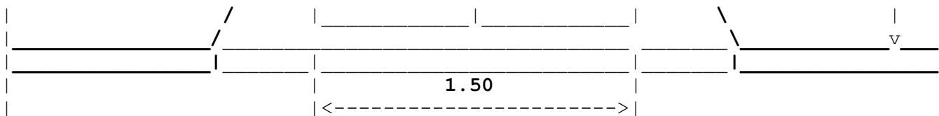
Fig. IV.8. - Rampă de acces între trotuar și carosabil
