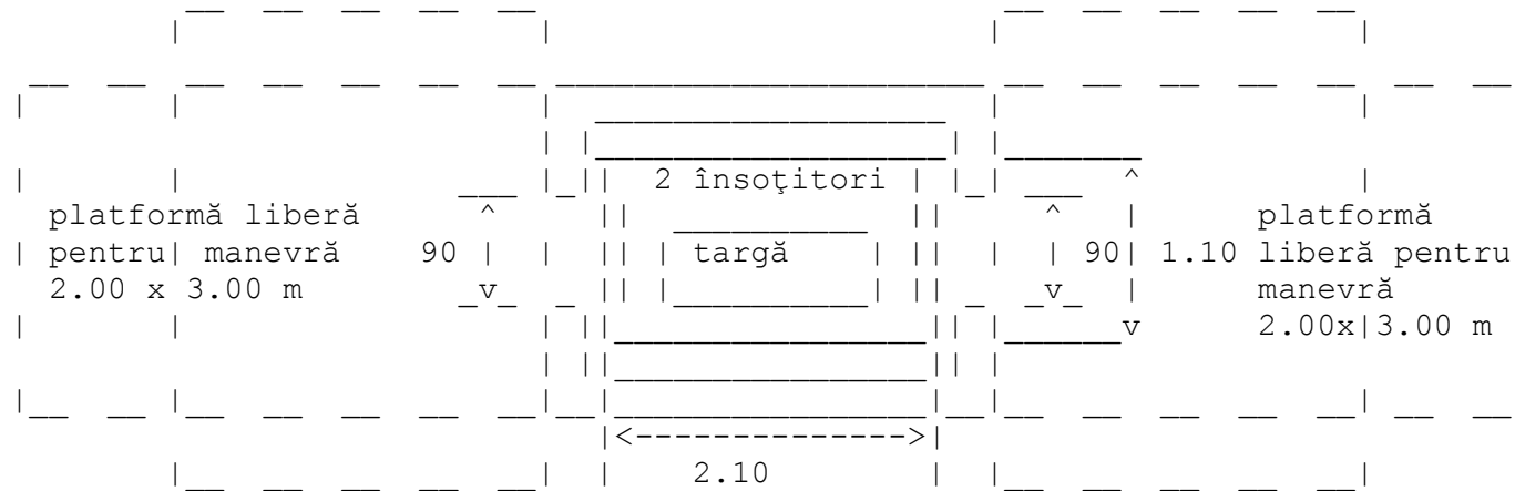
Fig. V.16. - Ascensor pentru transportul cu targa
