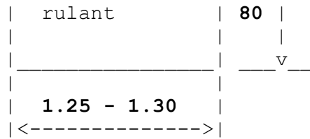
Fig. III.4. - Dimensiuni antropometrice minime pentru utilizatori ai fotoliului rulant - persoane adulte
