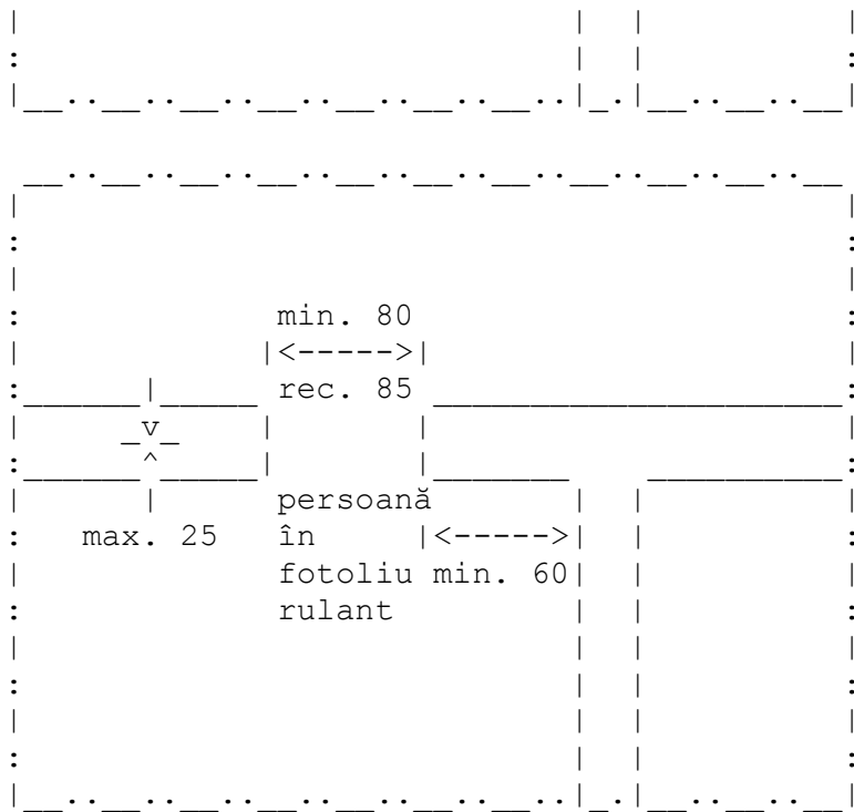
Fig. V.19. - Uși cu deschidere pe balamale sau pivot
